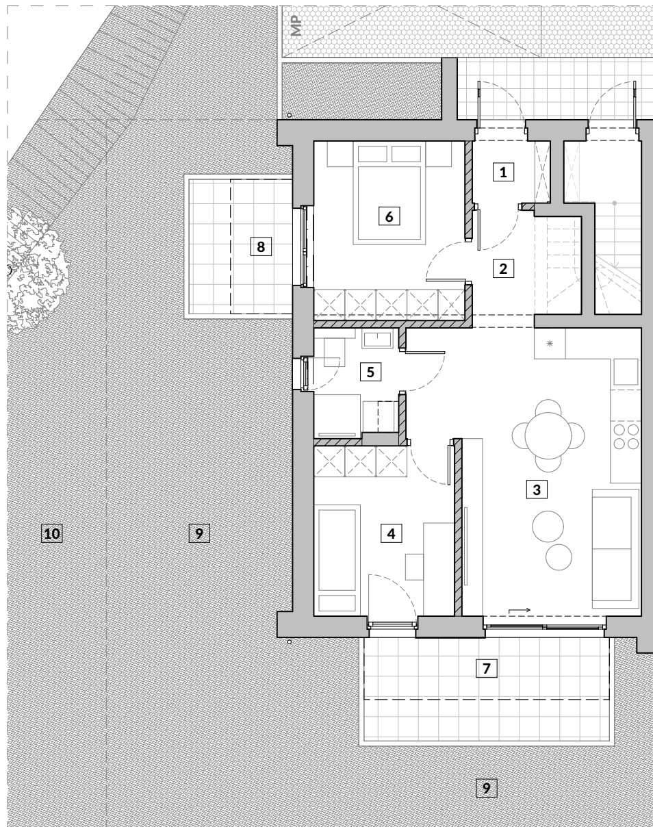
rzut parteru
